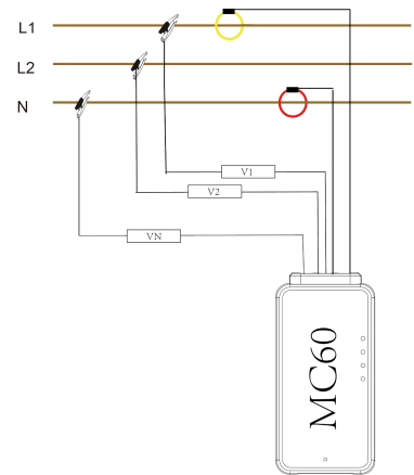
3P3W_2CT
