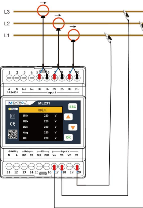
3P3W_3CT
