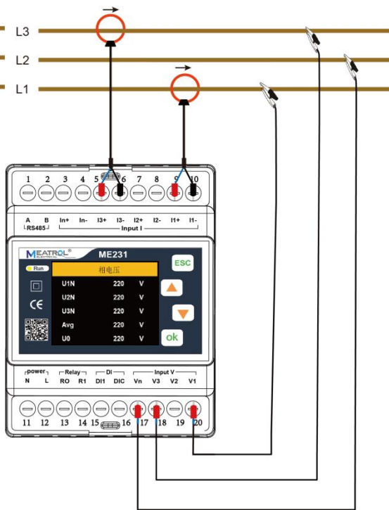
3P3W_2CT
