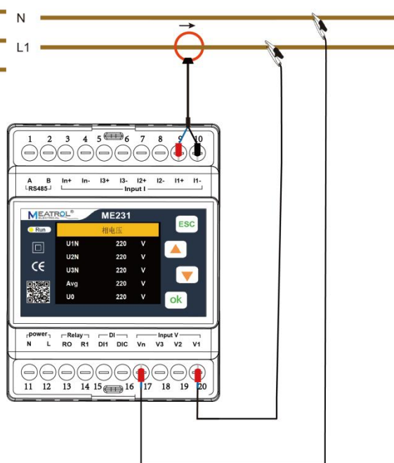
1P2W
