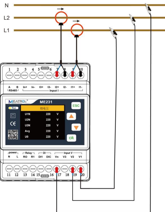
1P3W
